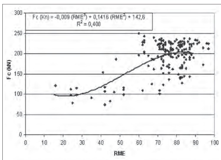
[Figura 8]- Correlación entre el RME y el empuje por cortador aplicado en la cabeza de corte.
